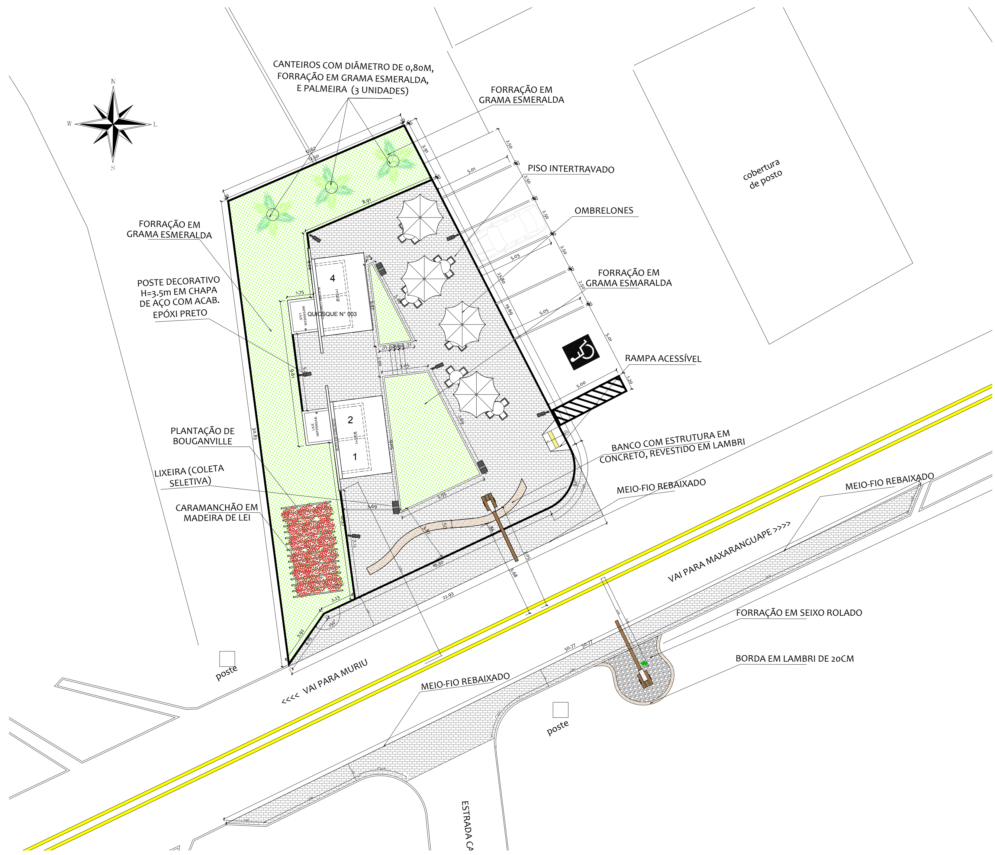
PLANTA DE LOCAÇÃO PÓRTICO E QUIOSQUE - MAXARANGUAPE Escala:..... 1/1 25
